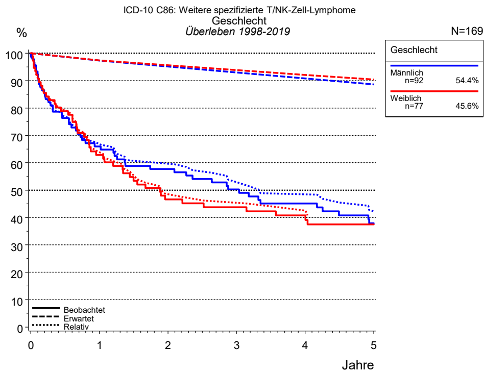
Abb. 2a. Beobachtetes, erwartetes und relatives Überleben für Patienten mit Weitere spezif. T/NK-Zell-Lymphome nach Geschlecht. In der Auswertung befinden sich 169 Patienten aus den Diagnosejahrgängen 1998 bis 2019.
