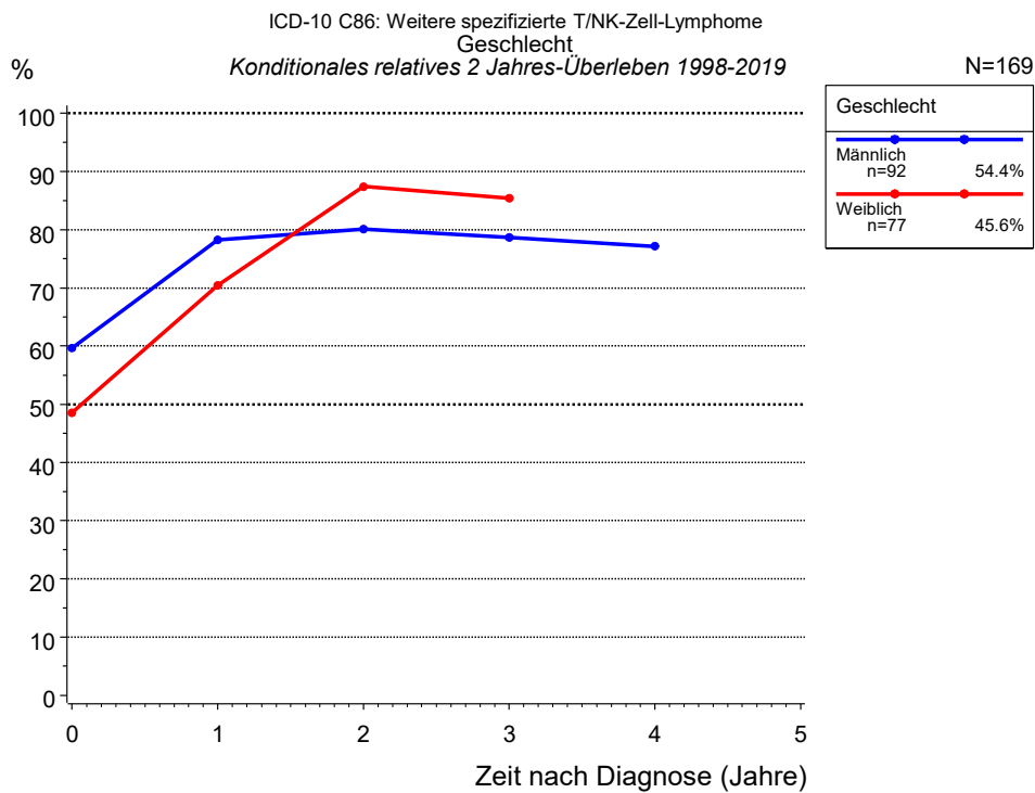
Abb. 2c. Konditionales relatives 2 Jahres-Überleben für Patienten mit Weitere spezif. T/NK-Zell-Lymphome nach Geschlecht. 169 von 169 Patienten aus den Diagnosejahrgängen 1998 bis 2019 besitzen Angaben zu diesem Merkmal.
