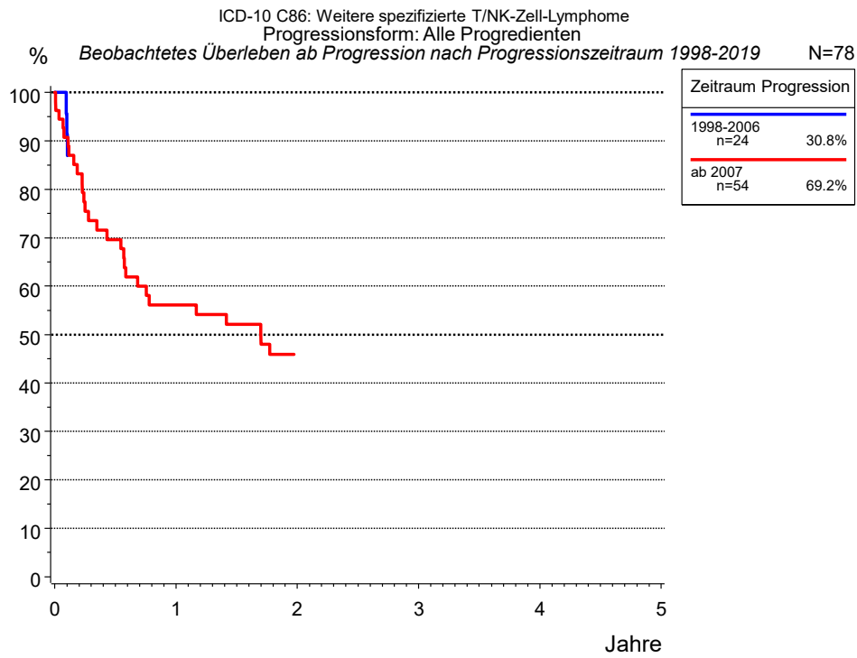
Abb. 5e. Beobachtetes Überleben ab erster Progression (Alle Progredienten) für 78 Patienten mit Weitere spezif. T/NK-Zell-Lymphome aus den Diagnosejahrgängen 1998 bis 2019 nach Zeitraum Progression.
