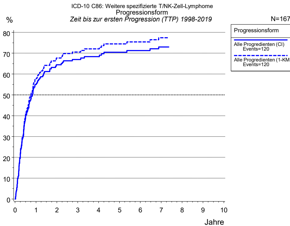
Abb. 5a. Zeit bis zum ersten Progressionsereignis für 167 Patienten mit Weitere spezif. T/NK-Zell-Lymphome aus den Diagnosejahrgängen 1998 bis 2019 (bei soliden Tumoren nur M0) geschätzt als kumulative Inzidenzfunktion (CI, durchgezogene Linie) mit Tod als konkurrierendes Risiko und als umgekehrter Kaplan-Meier-Schätzer (1-KM, gestrichelte Linie). Die Häufigkeit der Ereignisse kann aufgrund von Untererfassung unterschätzt sein.
