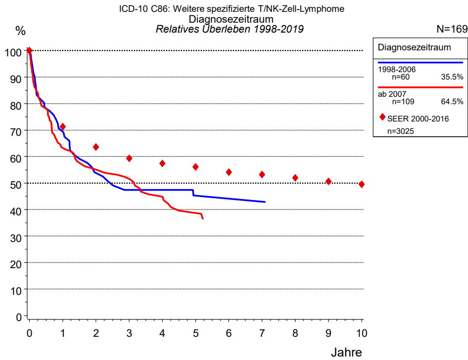
Abb. 1a. Relatives Überleben für Patienten mit Weitere spezif. T/NK-Zell-Lymphome nach Diagnosezeitraum. In der Auswertung befinden sich 169 Patienten aus den Diagnosejahrgängen 1998 bis 2019.
