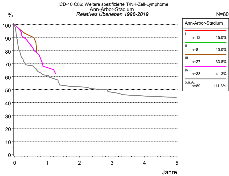
Abb. 4c. Relatives Überleben für Patienten mit Weitere spezif. T/NK-Zell-Lymphome nach Ann-Arbor-Stadium. 80 von 169 Patienten aus den Diagnosejahren 1998 bis 2019 besitzen Angaben zu diesem Merkmal. Die graue Linie repräsentiert 89 Patienten ohne auswertbare Angaben zum Merkmal Ann-Arbor-Stadium (52,7 % von 169 Patienten, die übrigen Prozentangaben beziehen sich auf n=80). Untergruppen mit Fallzahlen <20 sind nicht in der Grafik aufbereitet.
