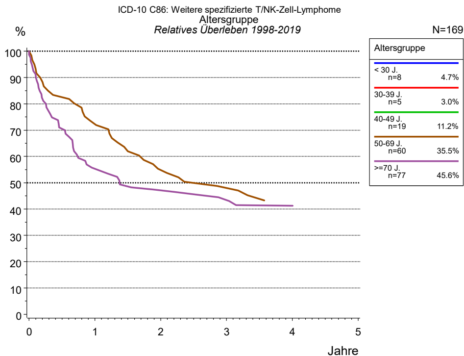
Abb. 3a. Relatives Überleben für Patienten mit Weitere spezif. T/NK-Zell-Lymphome nach Altersgruppe. In der Auswertung befinden sich 169 Patienten aus den Diagnosejahrgängen 1998 bis 2019. Untergruppen mit Fallzahlen <20 sind nicht in der Grafik aufbereitet.
